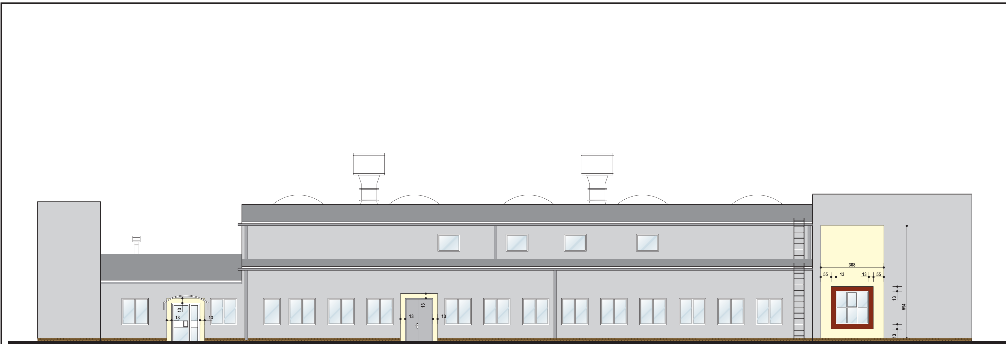
ELEWACJA POLUDNIOWO - ZACHODNIA
