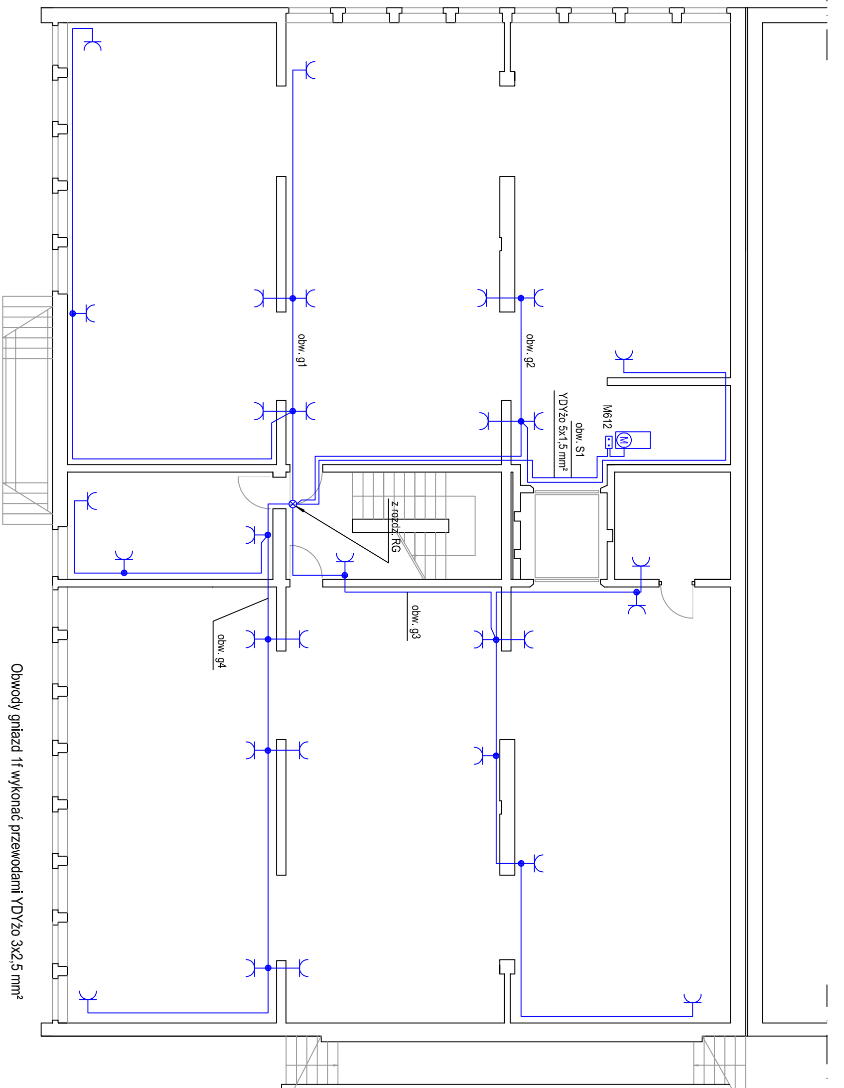
Układ sieci TN-C-S
